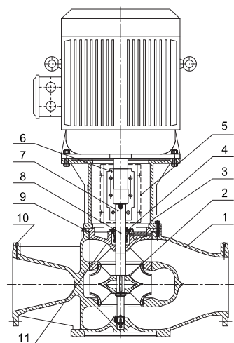
TD300材料表
