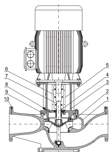
TD200-TD250材料表
