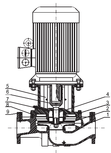
TD32-TD150材料表
